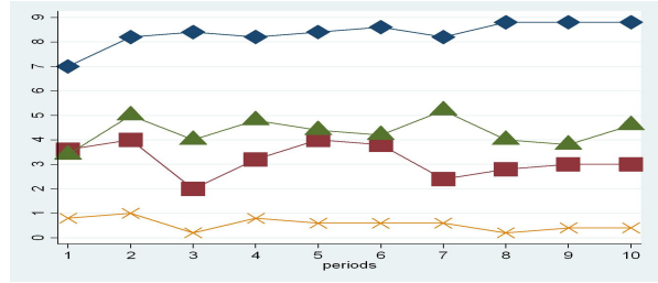
(d) Effort-Exclusion (2.2)
